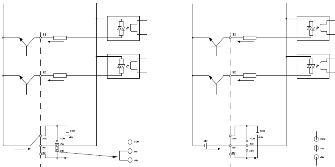
Режим с общим эмиттером (0V общий) для внутр. питания
