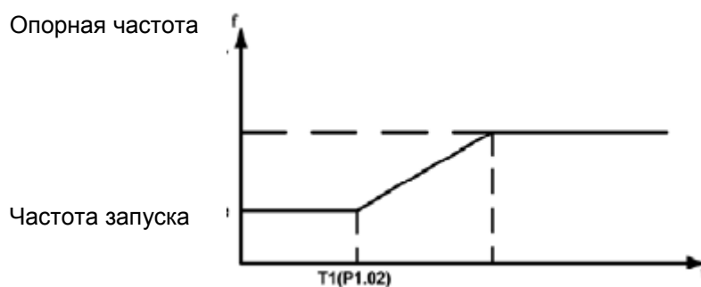
Рисунок 6.3. График пуска
